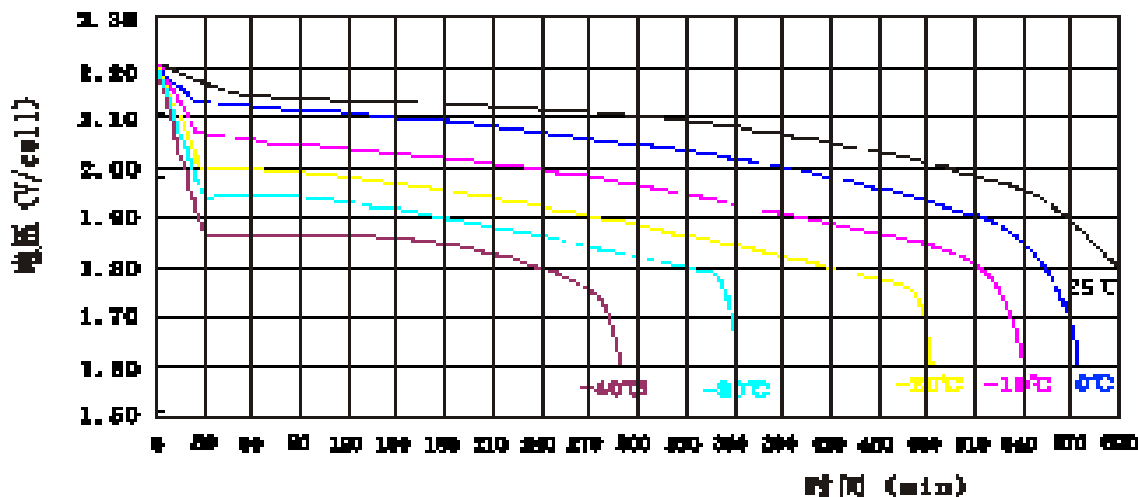
铅晶电池不同温度下放电曲线
